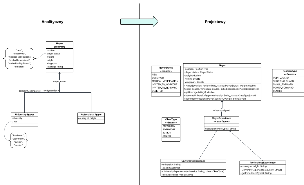
Rysunek 17: Fragment zmiany klas z analitycznego na projektowy diagram klas - Player, interfejs PlayerExperience oraz implementacje
