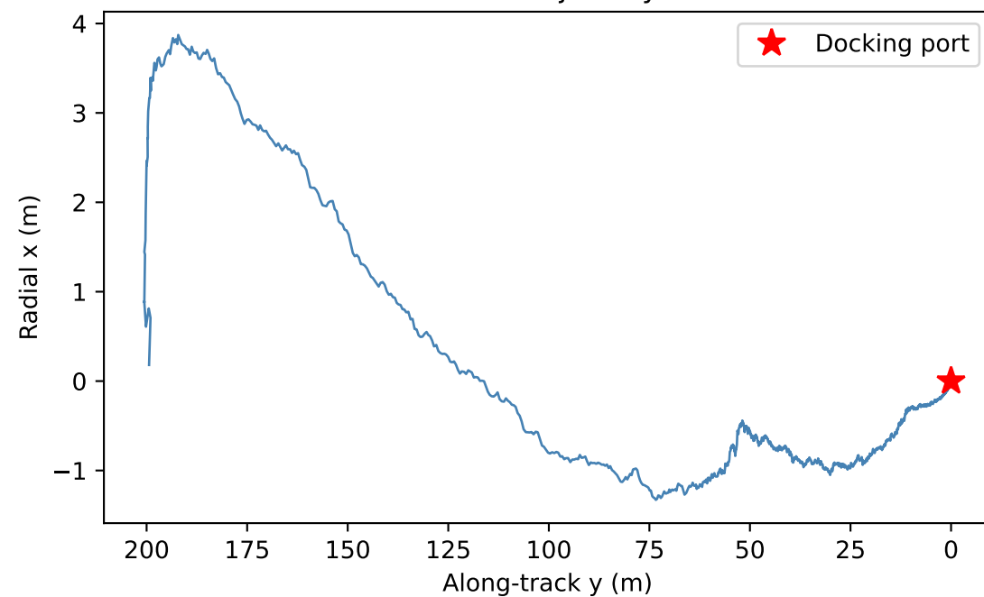
LVLH Trajectory
