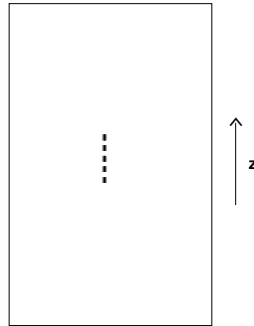
Imagen de la cuantificación canónica
