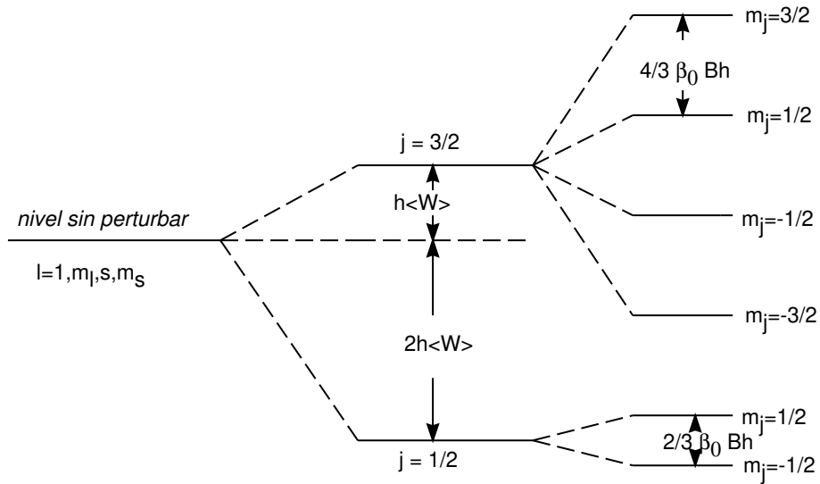
Estructura Fina Zeeman
