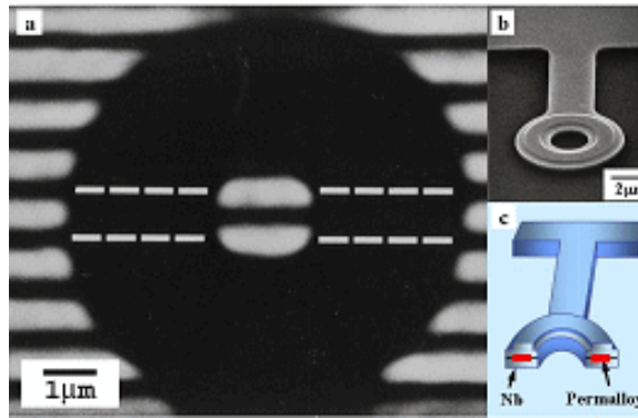
Figura 3: En el cuadro (a), se ve el anillo negro del magneto recubierto por el superconductor. En el orificio interior se ve como la línea de interferencia está desplazada respecto de las exteriores en una fracción de 1/2 . En los cuadros (b) y (c) se muestran detalles de la construcción del anillo.
