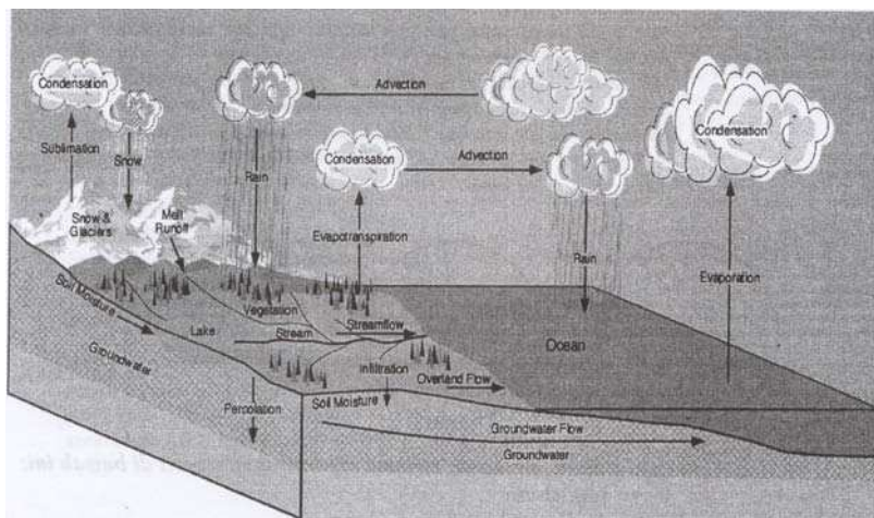
Gambar 6.8 Siklus Hidrologi
