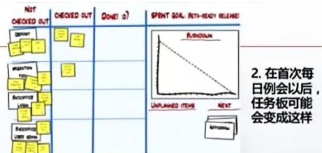
每日站会
