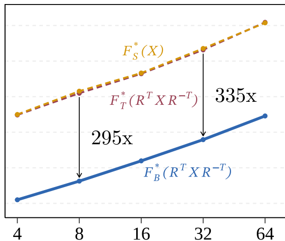
Matrix exp. adjoint
