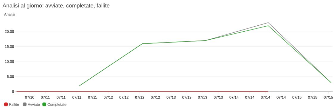
Figura 5: Analisi al giorno: avviate, completate e fallite (dati reali, CloudWatch). Lo scarto fra avviate e completate del 14/07 è un’analisi persa per il riavvio del container in modalità inprocess .
