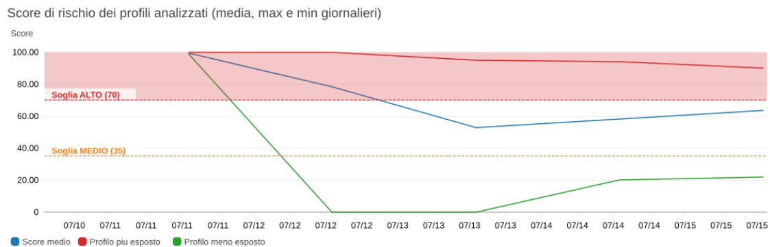
Figura 7: Score di rischio dei profili analizzati, con le soglie MEDIO (35) e ALTO (70) del modello.
