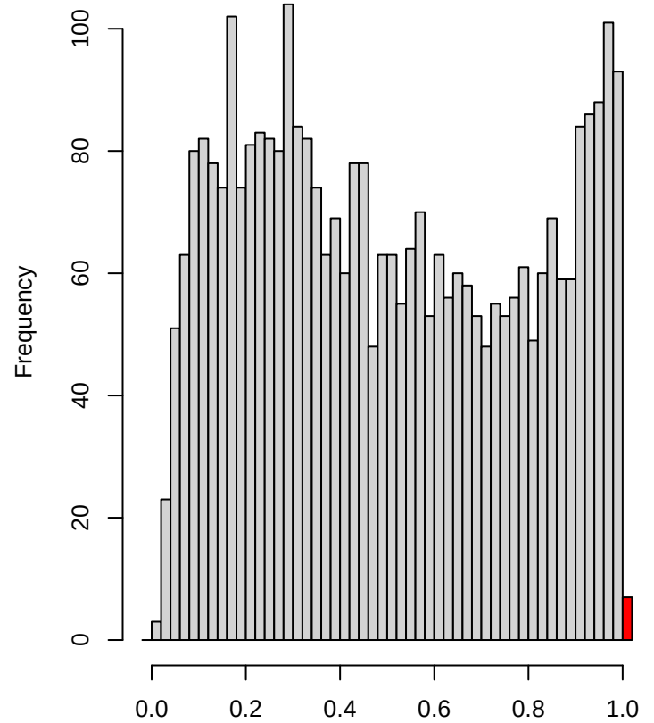
Outlier test n.s.
