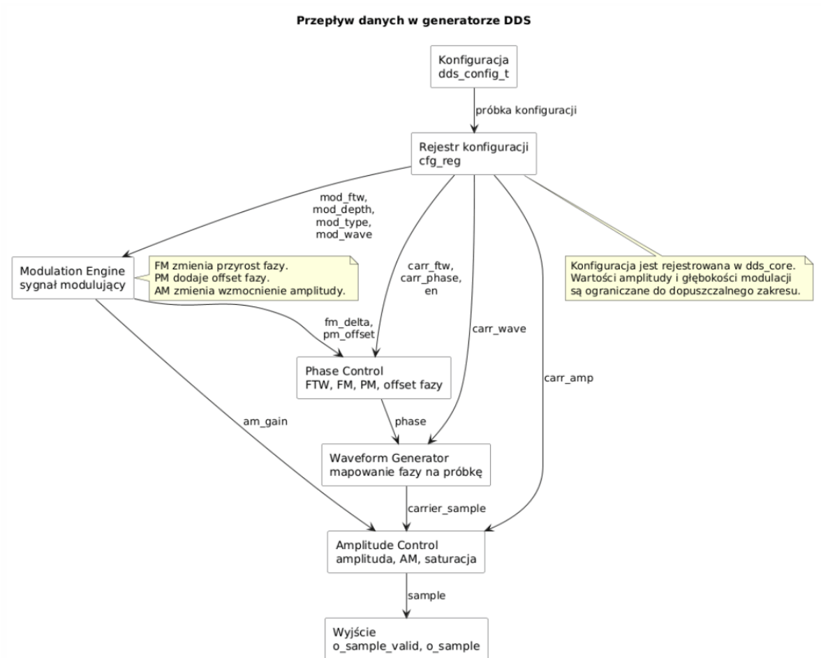
Rysunek 4.2: Przepływ danych w generatorze DDS.
