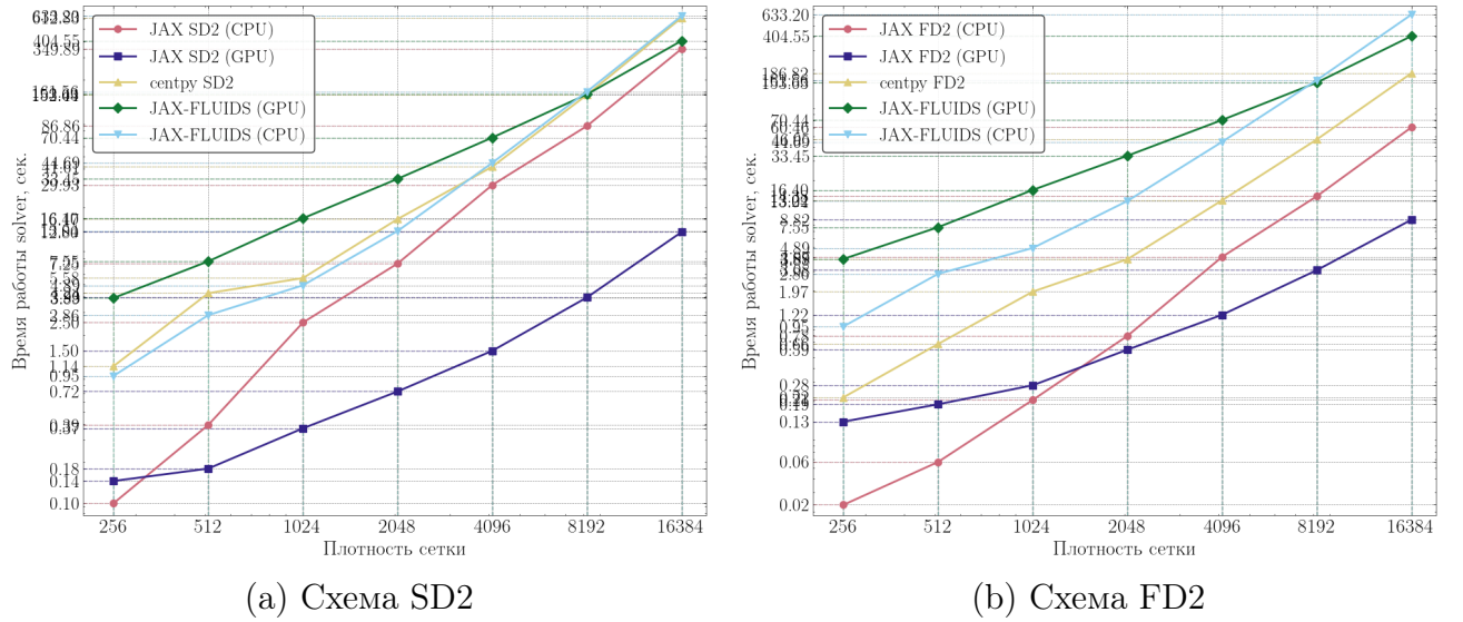
Рис. 17. Одномерная постановка. t_{\text{end}} = 0.4 , dt_{\text{out}} = 0.005 , CFL = 0.475 .
