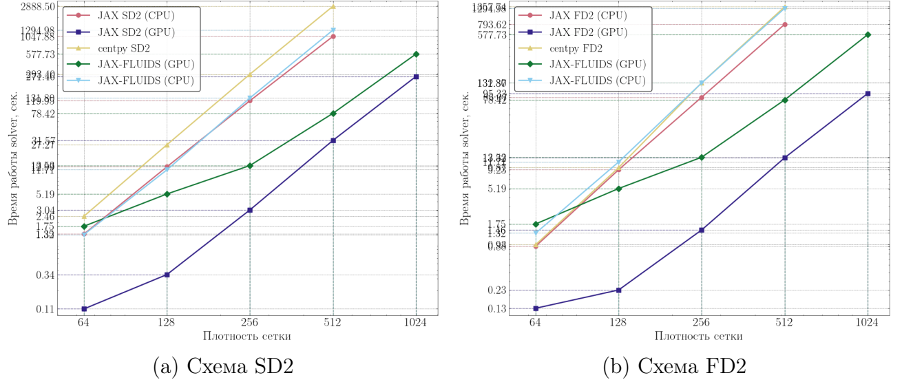
Рис. 18. Двумерная постановка. t_{\text{end}} = 0.4 , dt_{\text{out}} = 0.005 , \text{CFL} = 0.475 .
