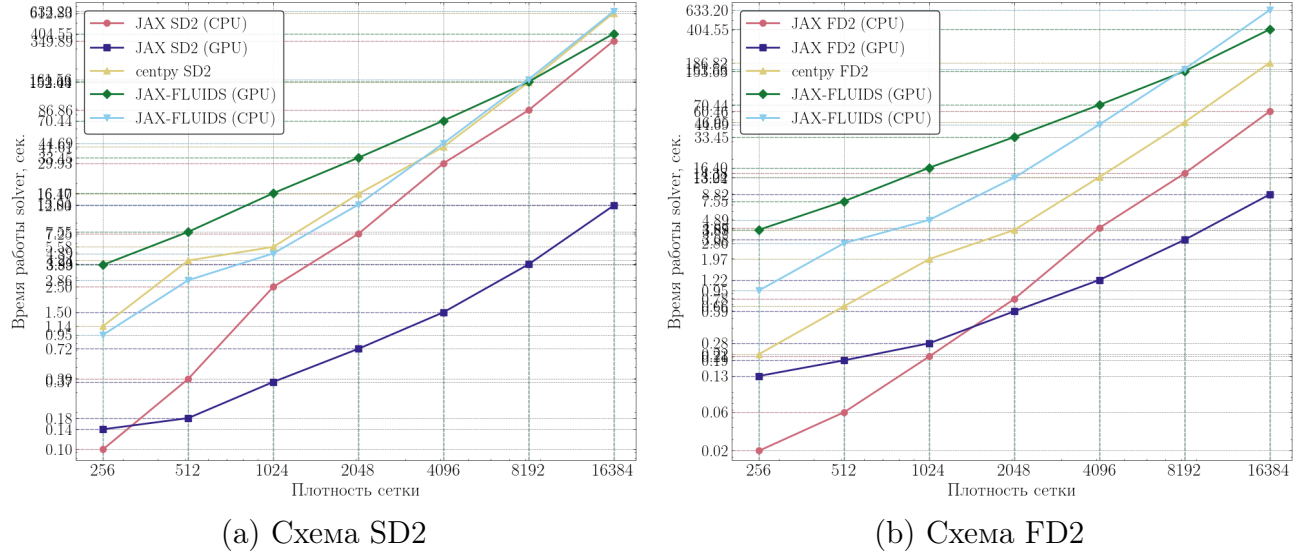
Рисунок 17. Одномерная постановка. t_{\text{end}} = 0.4 , dt_{\text{out}} = 0.005 , \text{CFL} = 0.475 .
