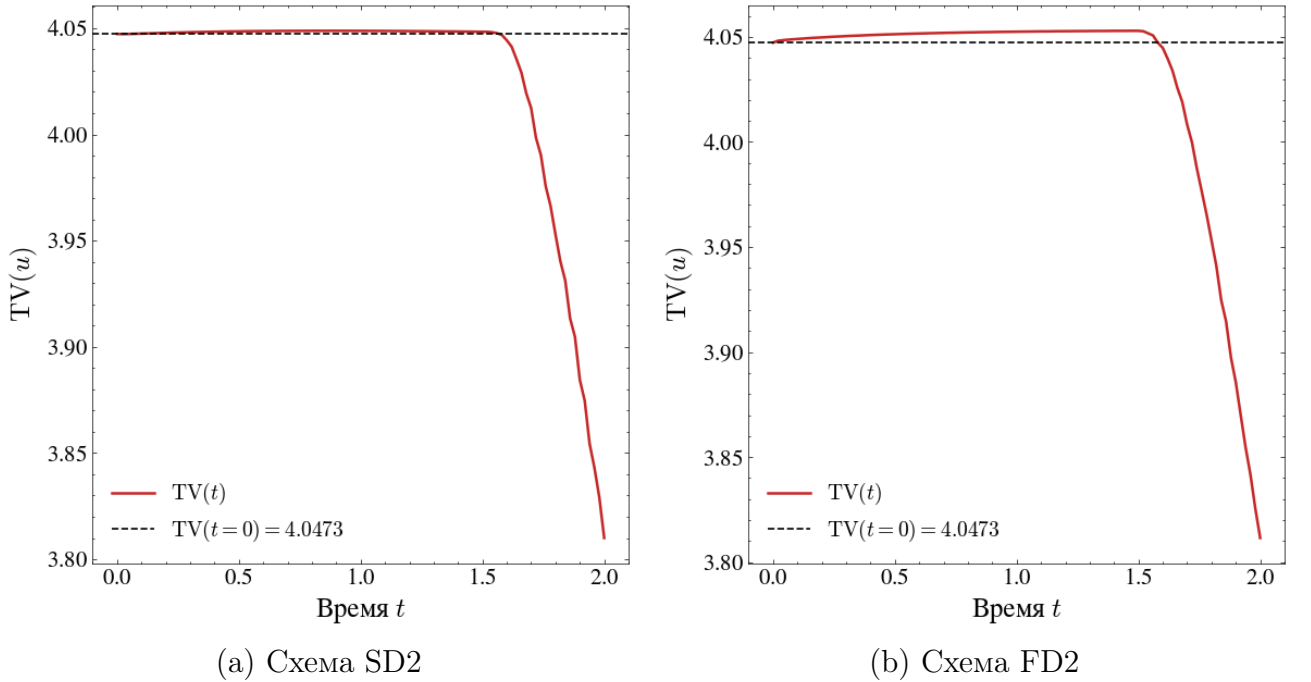
Рисунок 3. Эволюция полной вариации TV(t) для уравнения Бюргерса (83). Пунктирная линия соответствует начальному значению TV(t = 0) .
