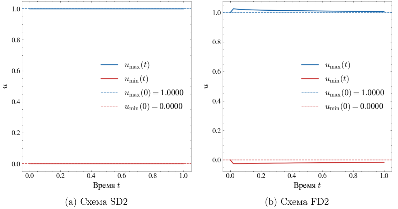
Рисунок 4. Эволюция u_{\min}(t) и u_{\max}(t) для задачи линейной адвекции (91). Пунктирные линии — начальные значения u_{\min}(t = 0) = 0 и u_{\max}(t = 0) = 1 .
