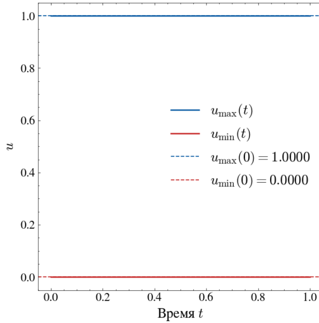
Рисунок 5. Эволюция u_{\min}(t) и u_{\max}(t) для задачи линейной адвекции (91). Схема FD2 , число Куранта C = 0.27
