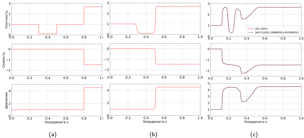
Рис. Эволюция примитивных переменных в модифицированной 1D задаче Римана (a) t = 0 ; (b) t = 0.125 ; (c) t = 0.25
