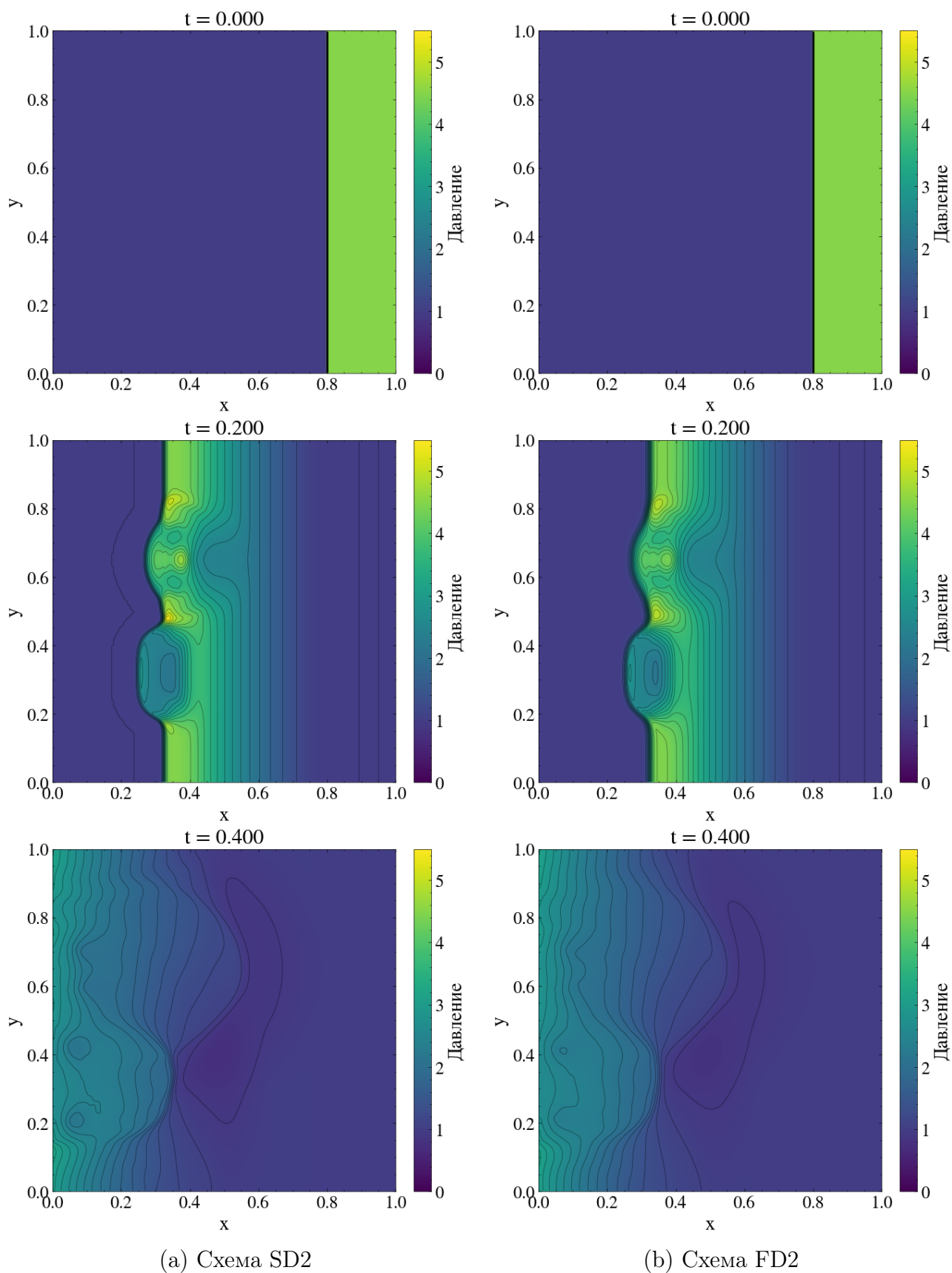
Рис. 11. Двумерная задача. Тепловые карты давления p(x, y) в три характерных момента времени.
