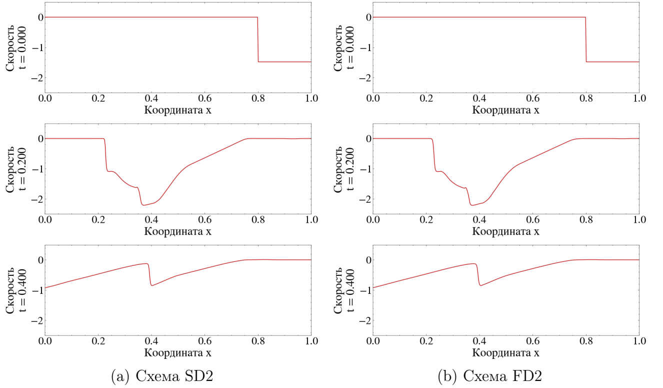
Рис. 7. Одномерная задача. Профили скорости u(x) в три характерных момента времени. Сетка N = 400 .
