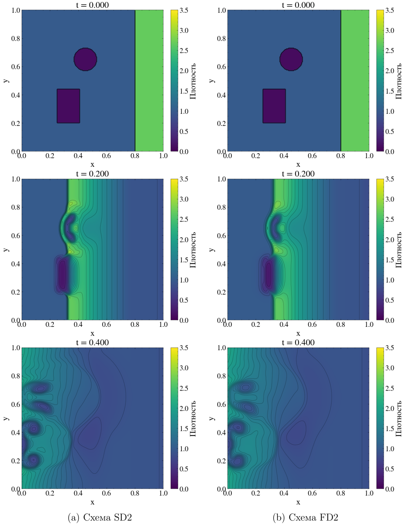
Рис. 9. Двумерная задача. Тепловые карты плотности \rho(x, y) в три характерных момента времени: t = 0 (начало), t = 0.2 (взаимодействие), t = 0.4 (завершение).
