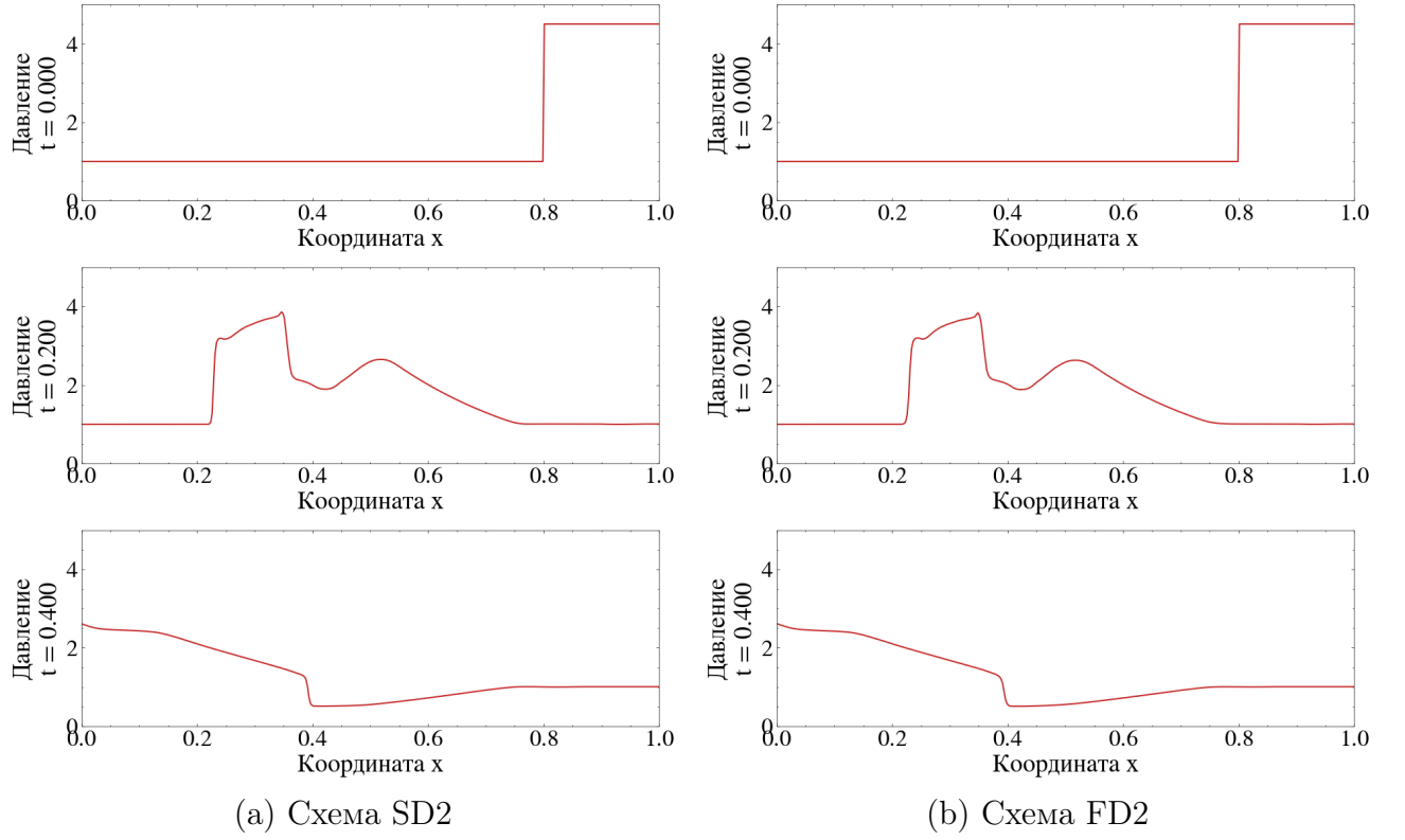
Рис. 8. Одномерная задача. Профили давления p(x) в три характерных момента времени. Сетка N = 400 .
