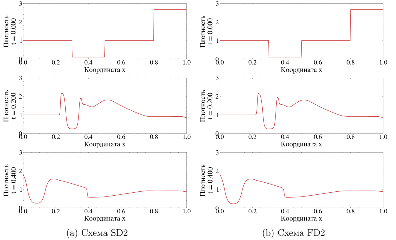
Рис. 6. Одномерная задача. Профили плотности \rho(x) в три характерных момента времени: t = 0 (начало), t = 0.2 (взаимодействие), t = 0.4 (завершение). Сетка N = 400 .
