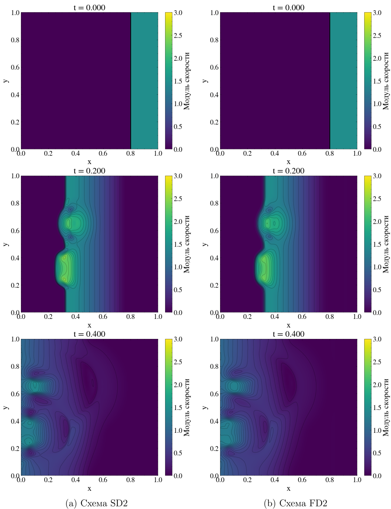
Рис. 10. Двумерная задача. Тепловые карты модуля скорости в три характерных момента времени.
