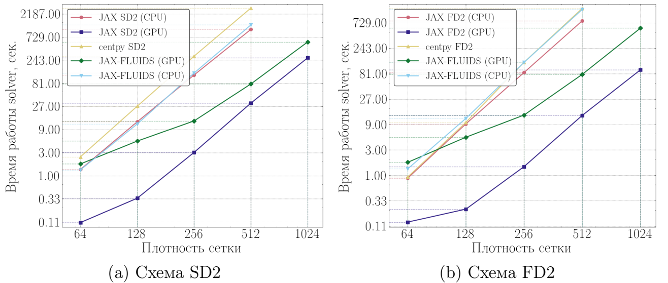
Рисунок 18 – Двумерная постановка. t_{\text{end}} = 0.4 , dt_{\text{out}} = 0.005 , \text{CFL} = 0.475
