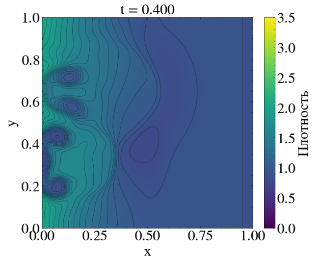
(b) Схема FD2
