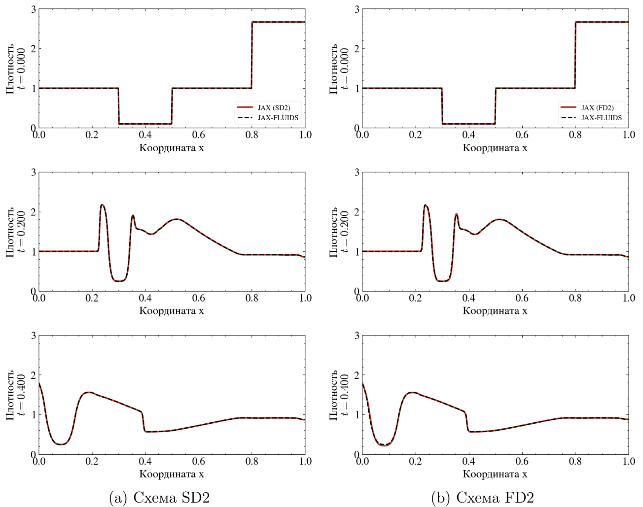
Рис. 12. Кросс-верификация параметра плотности относительно JAX-FLUIDS
