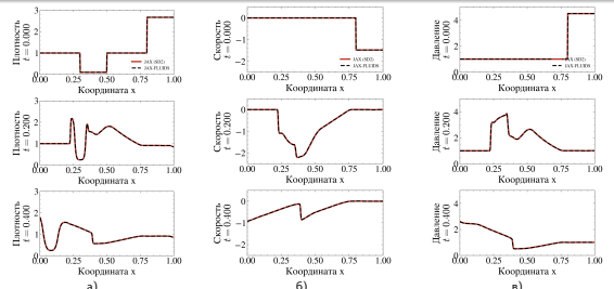
Рис. Эволюция примитивных переменных в модифицированной 1D задач Римана: а) плотность; б) скорость; в) давление (эталон JAX-FLUIDS)
