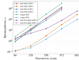
Рис. Время счета (с), 2D
