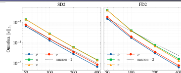
Рис. Ошибка по \rho, p, u, v в нормах L_1, 2D
