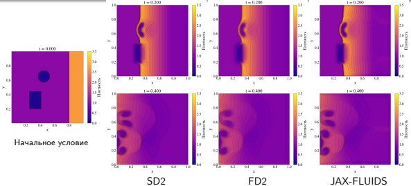
Рис. Эволюция плотности (эталон JAX-FLUIDS)
