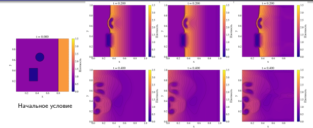
Рис. Эволюция плотности (эталон JAX-FLUIDS)
