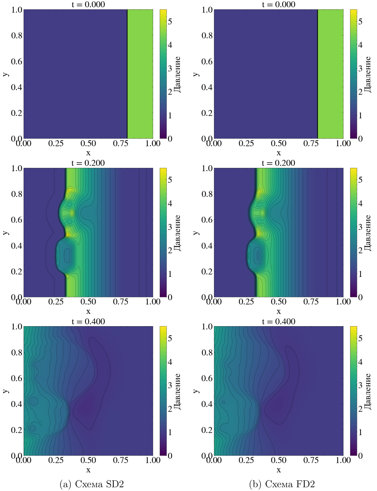
Рисунок 11 – Двумерная задача. Тепловые карты давления p(x, y) в три характерных момента времени: t = 0.0, 0.2, 0.4 . Параметры: Сетка 200 \times 200 , CFL = 0.475
