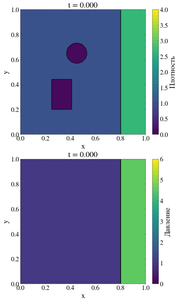
Рисунок 2 – Постановка модифицированной задачи в двумерном случае
