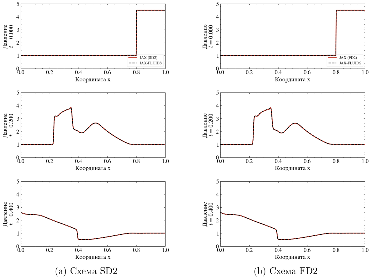
Рисунок 14. Кросс-верификация поля давления относительно JAX-FLUIDS
