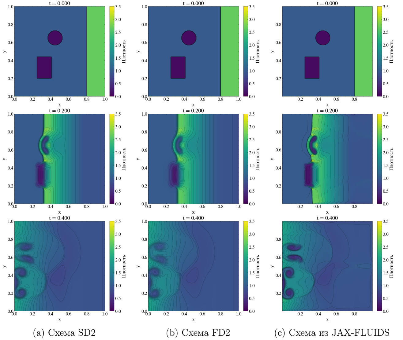
Рис. 16. Двумерная задача. Тепловые карты плотности p(x, y) в три характерных момента времени: t = 0.0, 0.2, 0.4 . Параметры: Сетка 200 \times 200 , CFL = 0.475 .
