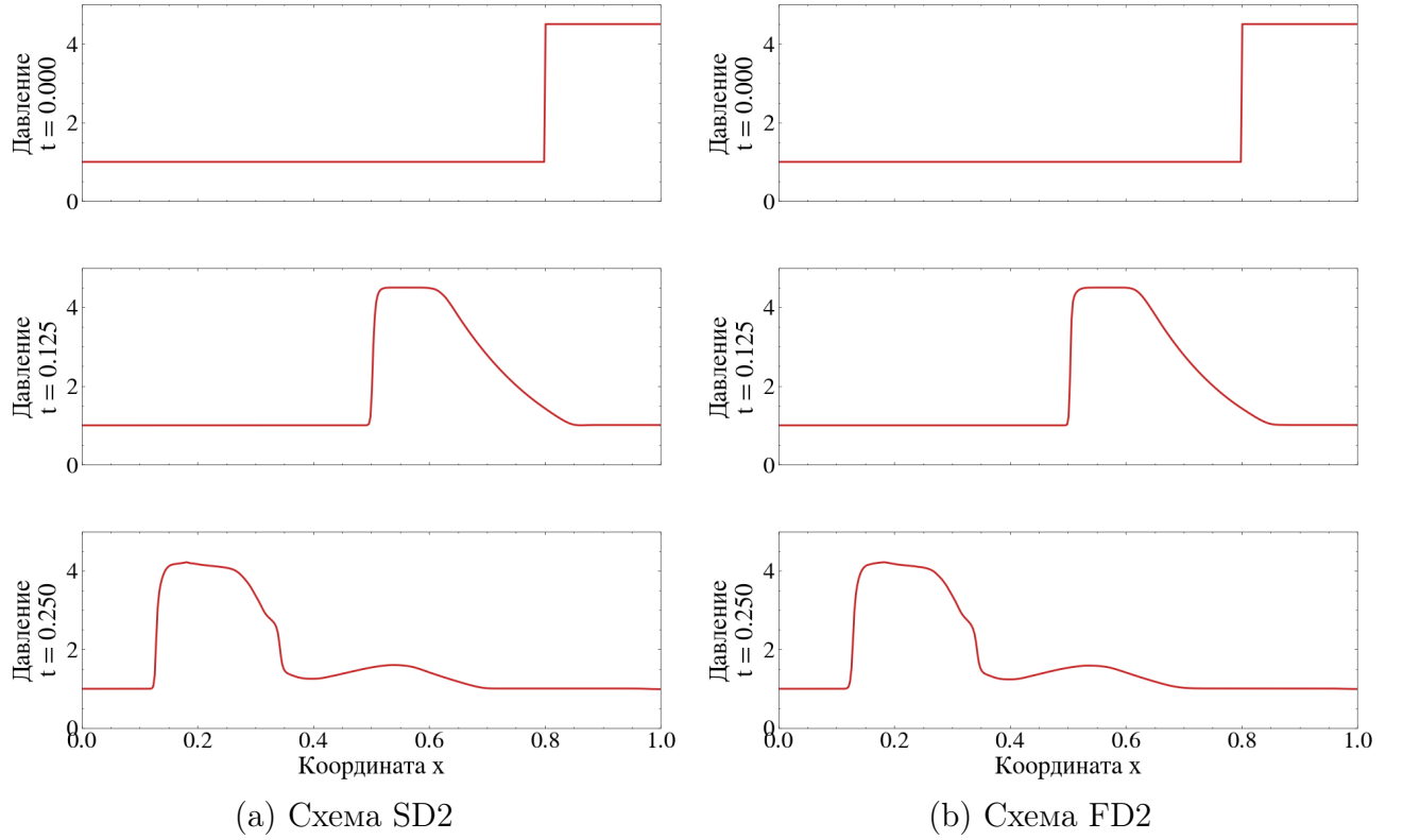
Рис. 8. Одномерная задача. Профили давления p(x) в три характерных момента времени. Лимитер minmod , N = 400 .
