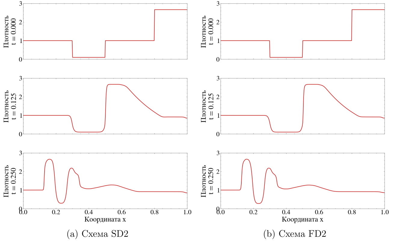
Рис. 6. Одномерная задача. Профили плотности \rho(x) в три характерных момента времени: t = 0 (начало), t = t_{1/2} (взаимодействие), t = t_{\text{end}} (завершение). имитер minmod , N = 400 .
