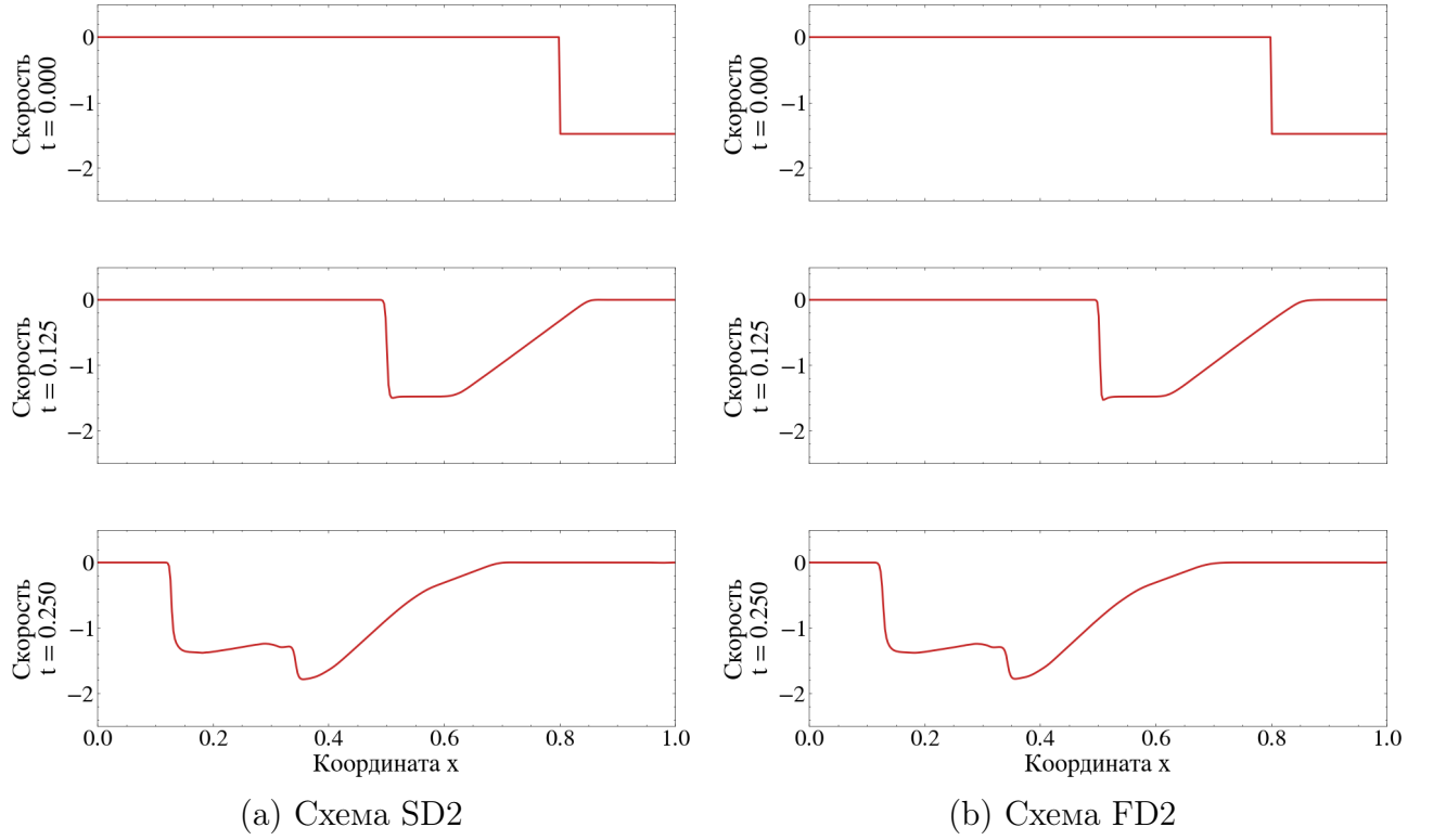
Рис. 7. Одномерная задача. Профили скорости u(x) в три характерных момента времени. Лимитер minmod , N = 400 .
