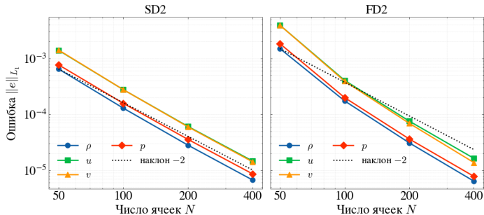
Рис. Ошибка по \rho, u, v, p , норма L_1 , 2D
