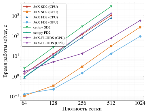
Рис. Время счёта (с) от размера сетки J \times J , 2D
