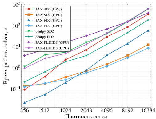
Рис. Время счёта (с) от размера сетки J , 1D
