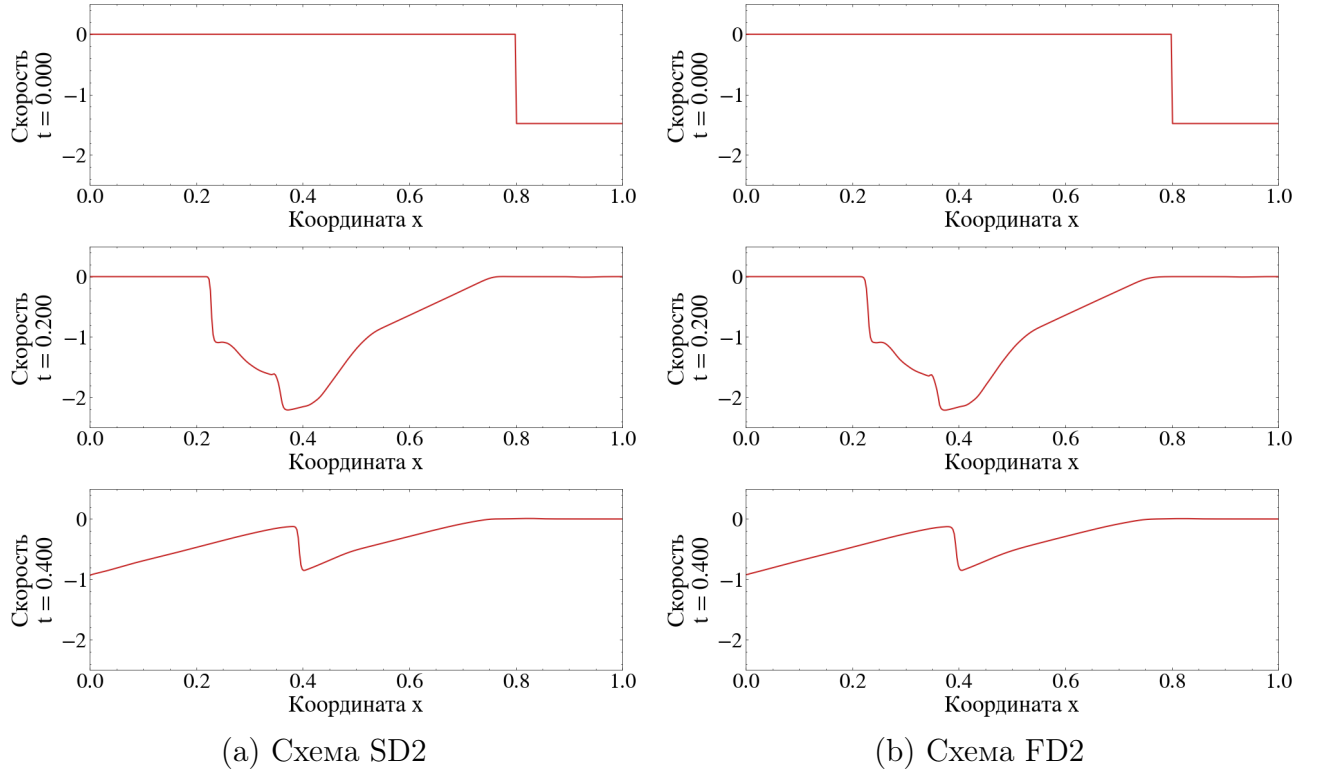
Рисунок 7. Одномерная задача. Профили скорости u(x) в три характерных момента времени: t = 0.0, 0.2, 0.4 . Параметры: N = 400 , CFL = 0.475 .
