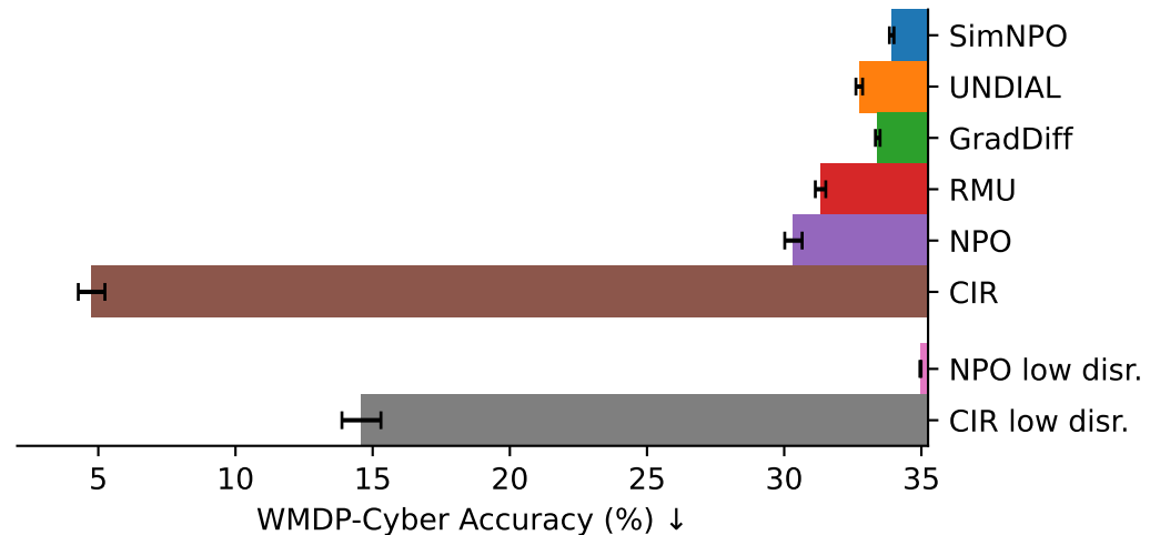
WMDP-Cyber
