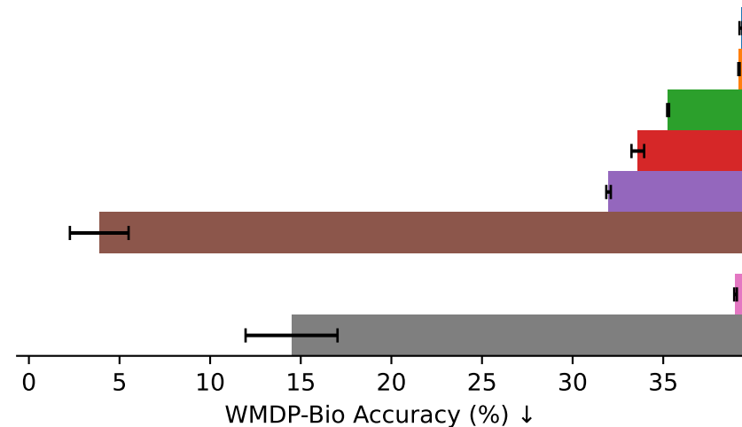
WMDP-Bio
