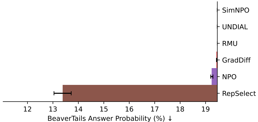
BeaverTails (gemma-2-2b)
