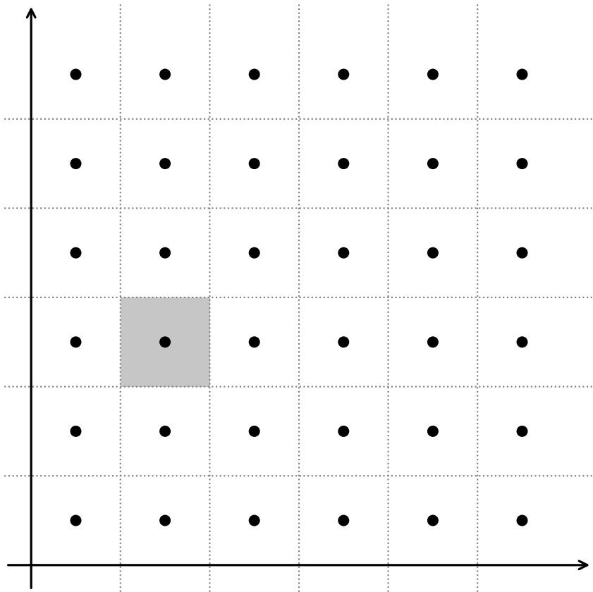
Центрированная решётка \Gamma_6^c в [0, 1]^2
