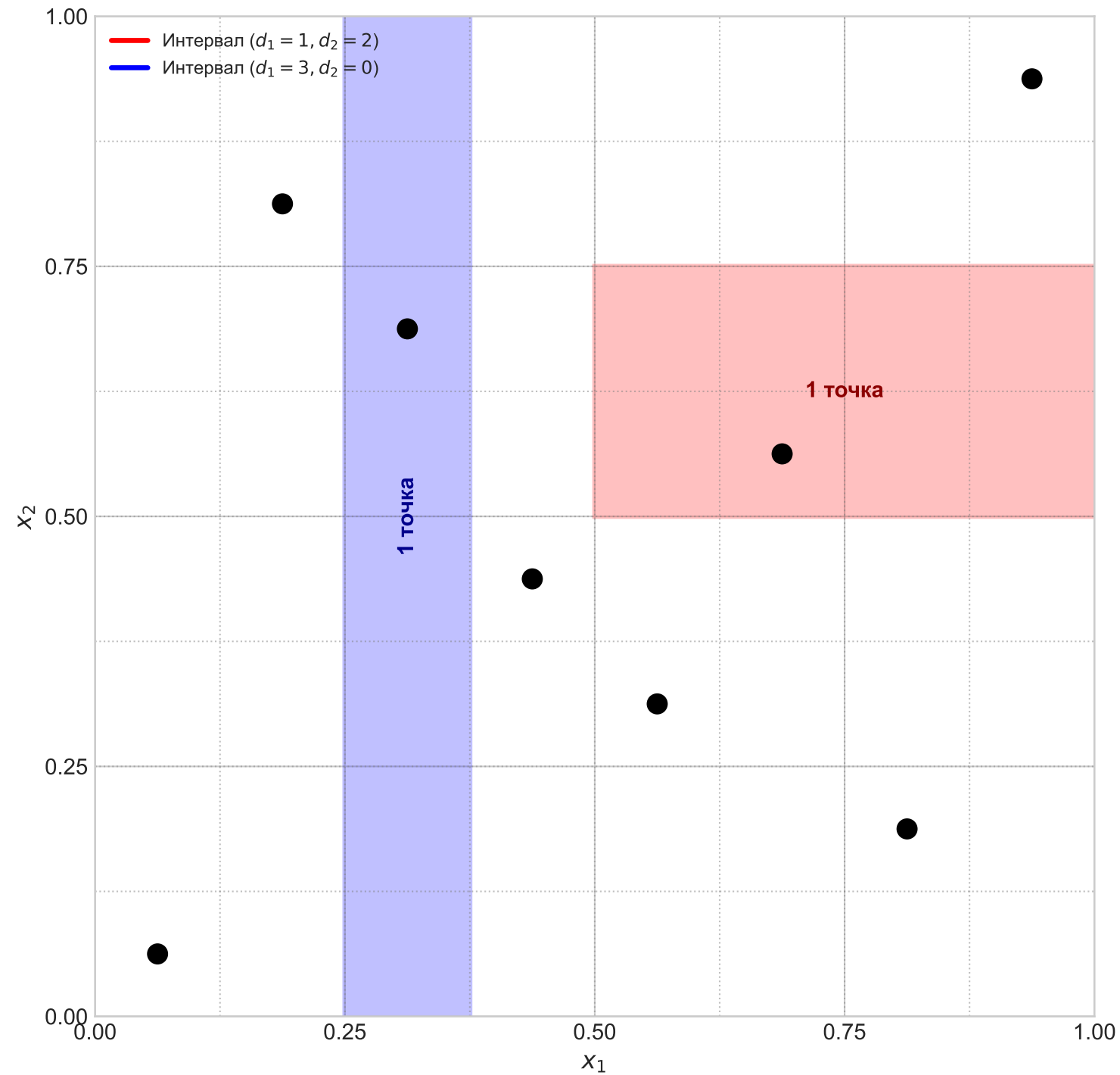
(0, 3, 2) -сеть в базе b = 2 (элементарные интервалы)
