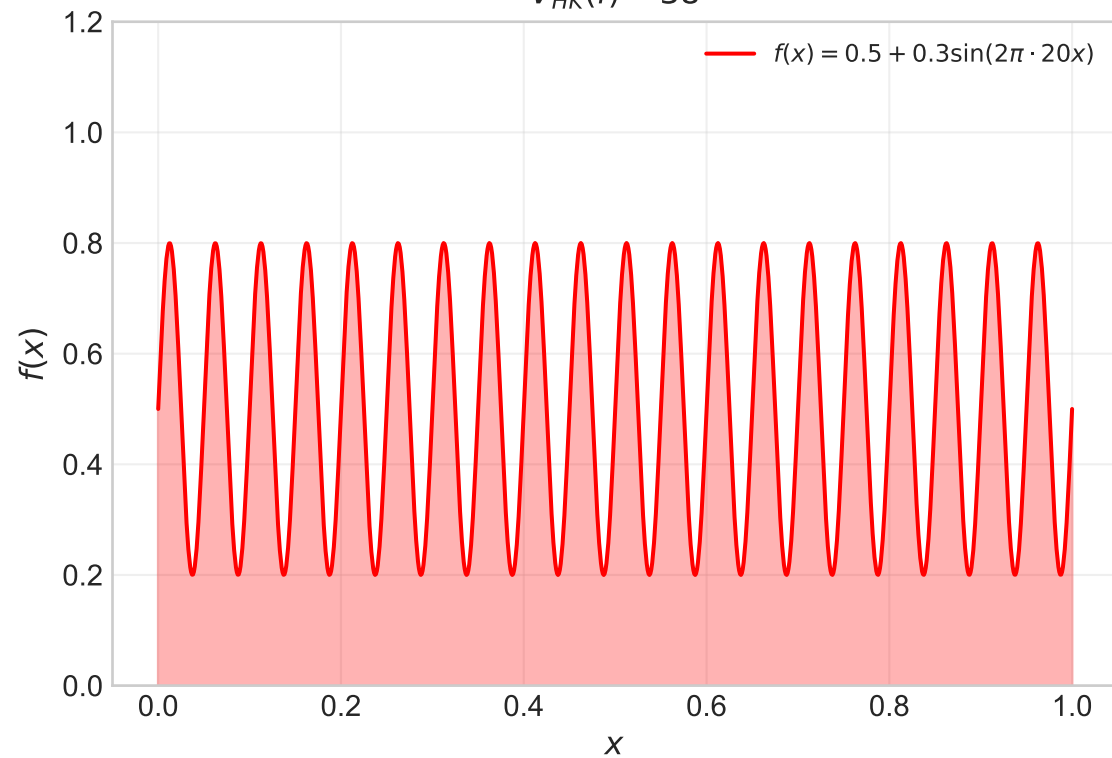
(b) Осциллирующая функция V_{HK}(f) \approx 38
