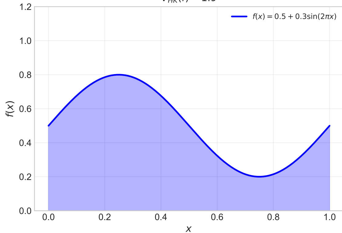
(a) Гладкая функция V_{HK}(f) \approx 1.9
