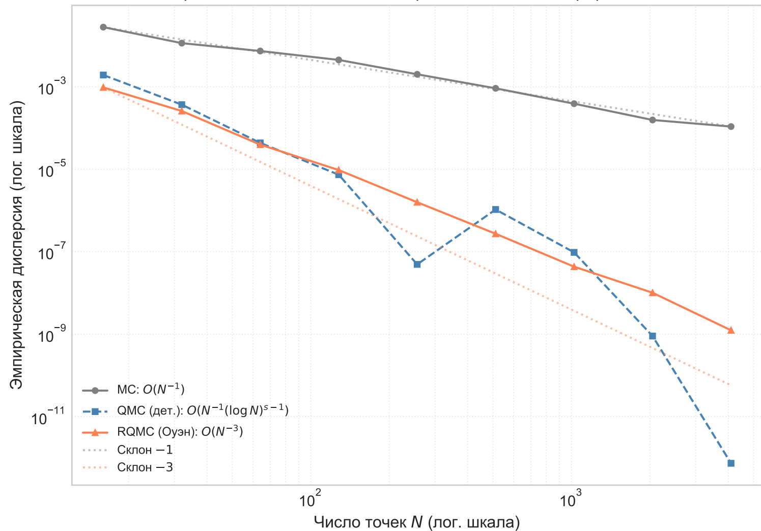
Сравнение сходимости дисперсии методов интегрирования
