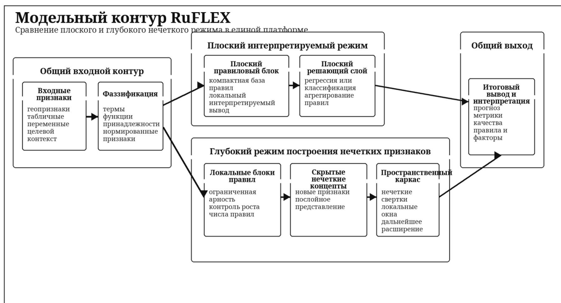
Рис. 2. Схема 2. Общий модельный контур RuFLEX с плоским и глубоким режимами.
