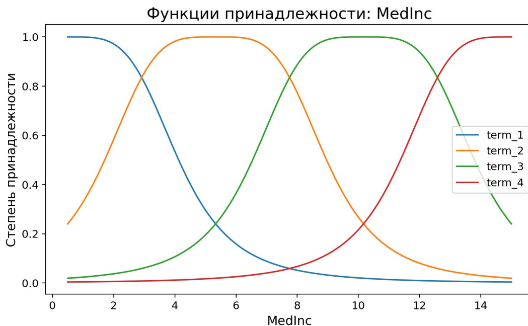
Рис. 8. Рис. 5. Пример функций принадлежности для интерпретируемой фазификации входного признака.
