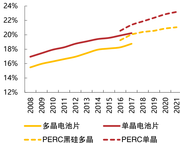
多晶与单晶电池片最高效率对比
