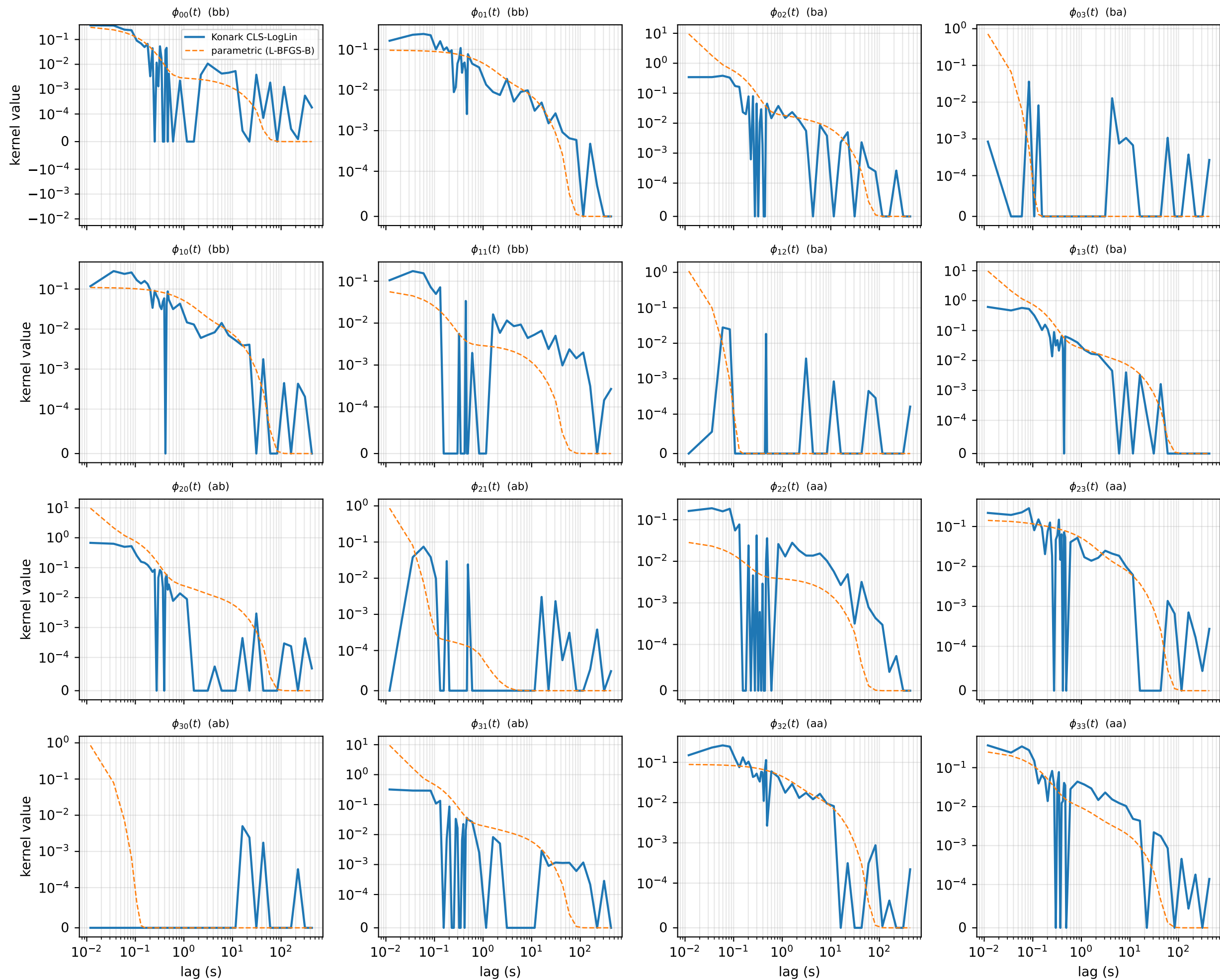
EUR/USD 2021-07-20: Konark CLS-LogLin kernel (4x4 grid) rho=0.9784 (vs EM 0.937, L-BFGS-B 0.988)
