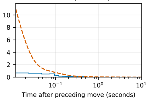
(d) Bid up \rightarrow Ask up
