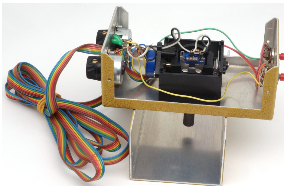
Рис. 5: A2D Joystick в разобранном виде
