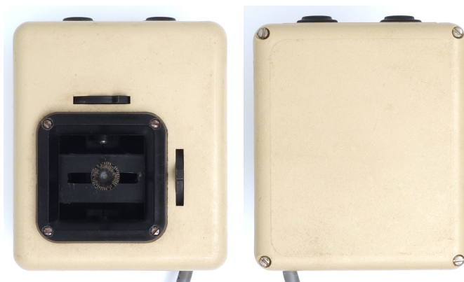
Рис. 2: A2D Joystick 2001, вид сверху и снизу
