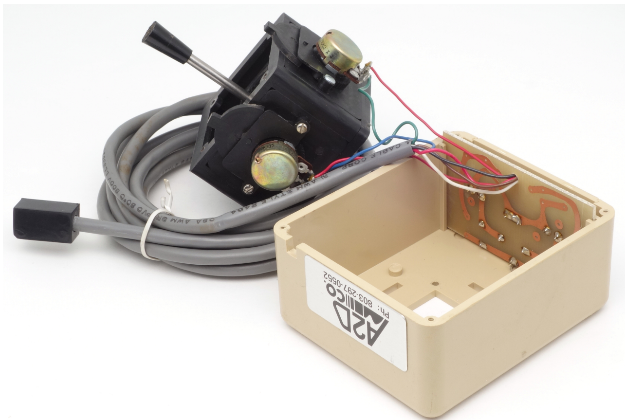
Рис. 6: A2D Joystick 2001 в разобранном виде
