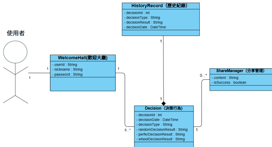
圖 2 領域模型
