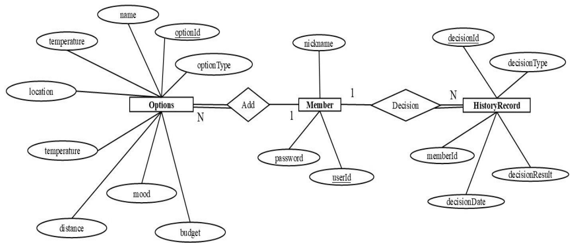
圖 3 ER Model
