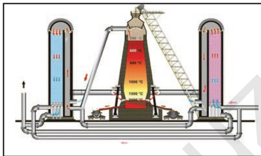
16- rasm. Domna pechlari tuzilishi.
