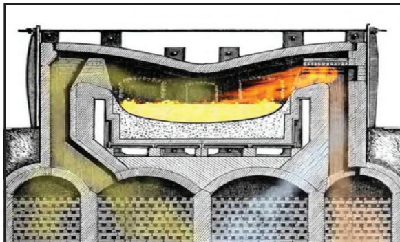
18- rasm. Marten pechi (kesmasi).
