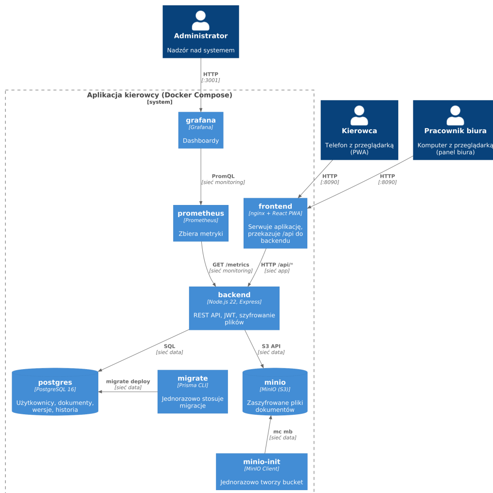
Rysunek 1: Diagram kontenerów systemu (model C4)
