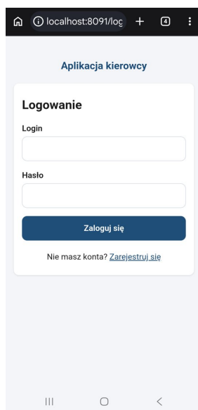
(a) logowanie
