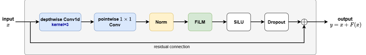
图 31: TCN 残差块架构。
