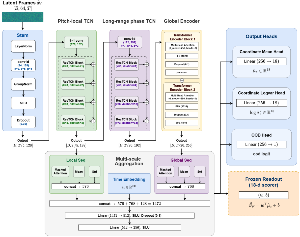
图 30: LTSN 架构图。
