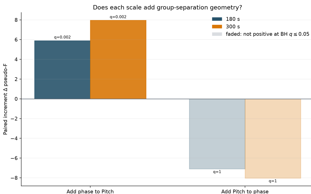
图 24: Pitch 与 Phase 的双向配对增量消融。只有 \Delta F > 0 且 BH-FDR q \leq 0.05 才判为正增量。
