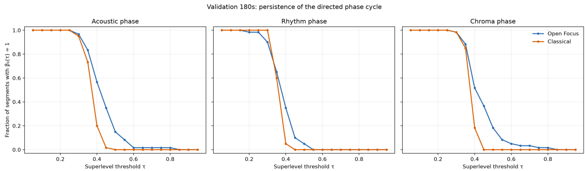
图 22: validation/180s 中完整六相位有向环在超水平阈值下的保留比例。该曲线是 loop_score 分布的路径同调表达，不作为独立统计证据。
