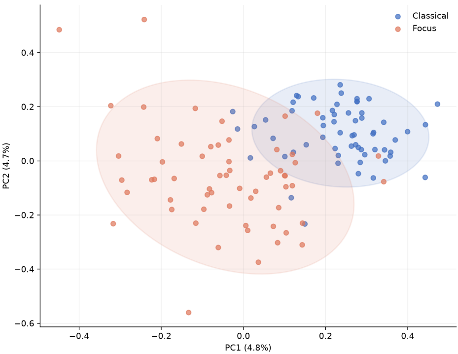
图 15: 由 discovery/180s 拟合的 PCA 对 validation/180s 三视角融合表示的二维投影。每个点代表一首曲目；椭圆阴影表示以组内均值为中心、沿组内协方差主轴延伸 1.96 个标准差的投影范围，并非 bootstrap 置信区间。
