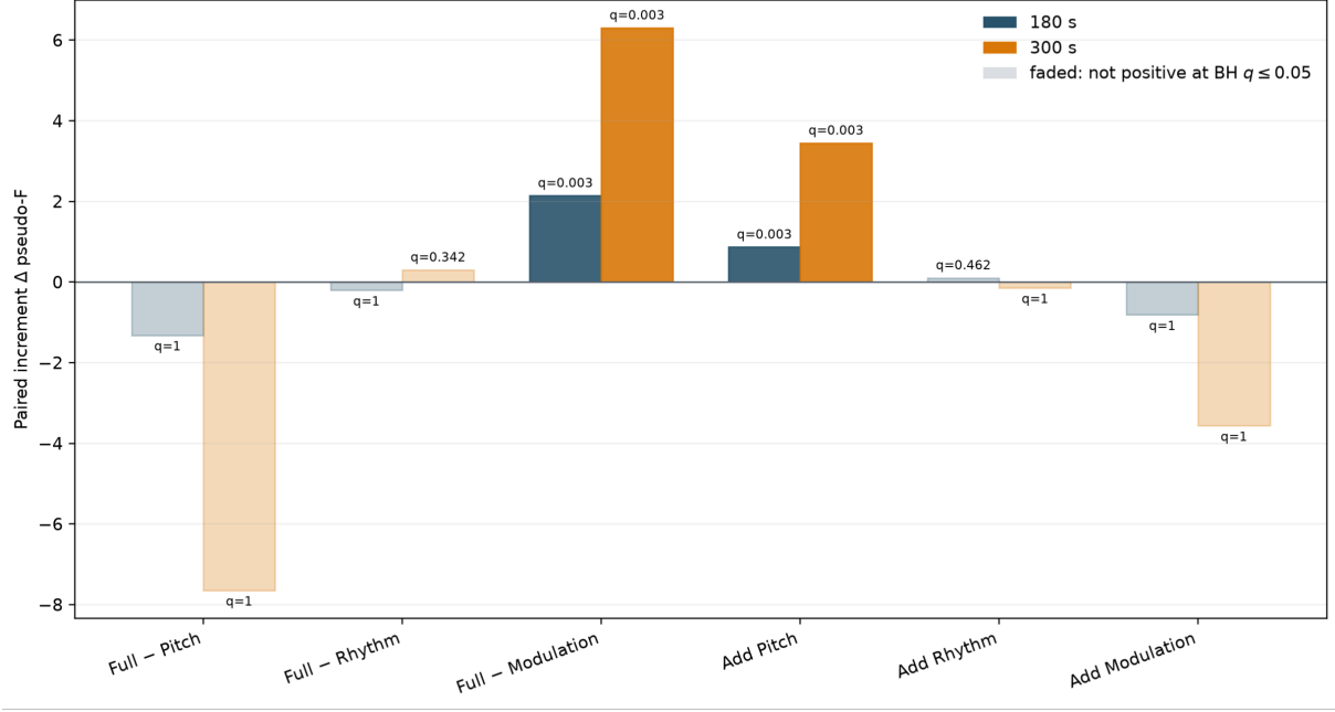
图 16: 局部三视角融合的对伪 F 增量检验。浅色柱表示未同时满足 \Delta F > 0 与 BH-FDR q \leq 0.05 ; 300s 仅作同曲目时长敏感性。
