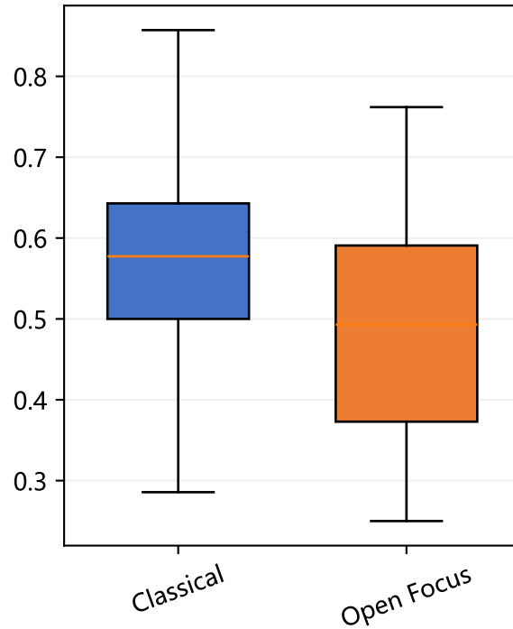
Edge density
