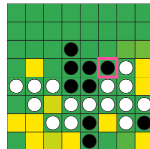
IM
