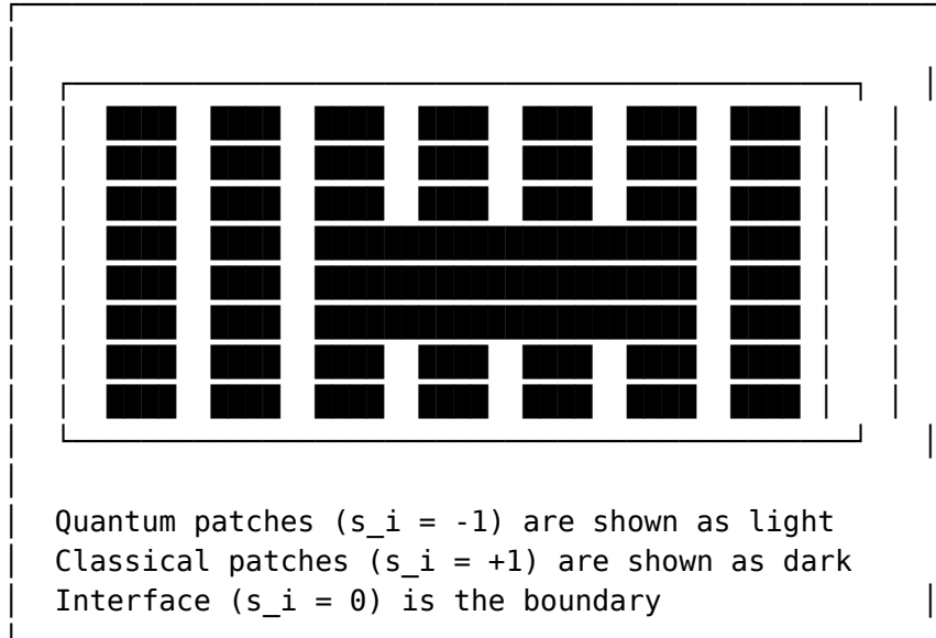
Figure N.1: Dynamic regime partitioning on the 2D lattice
