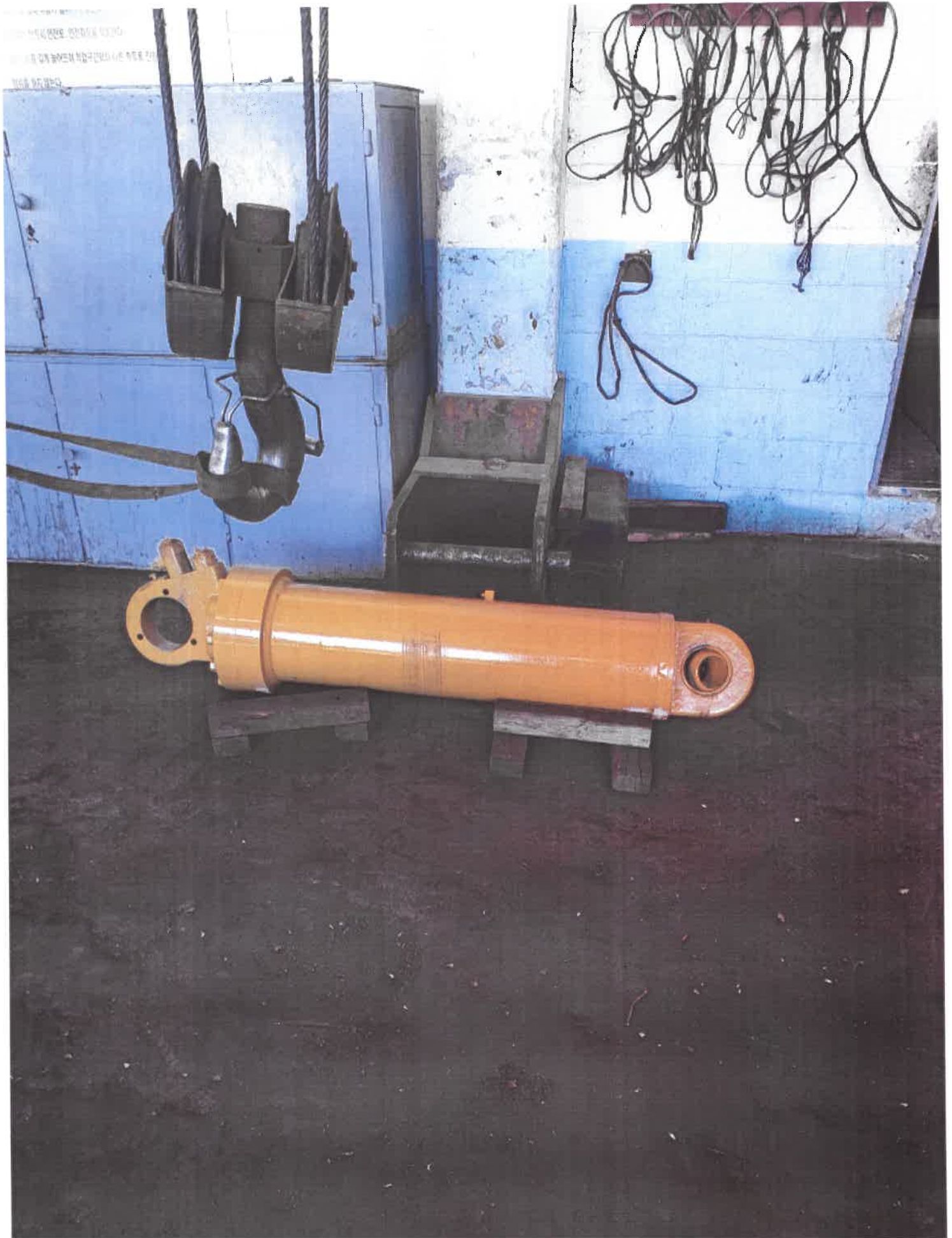
트랙 리프트실린더
