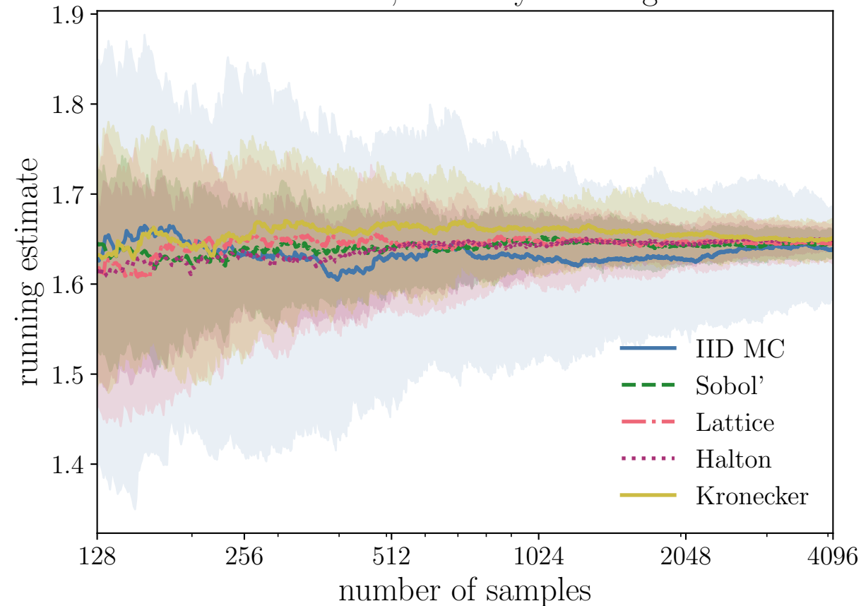
Posterior Gaussian, Cholesky: running estimates
