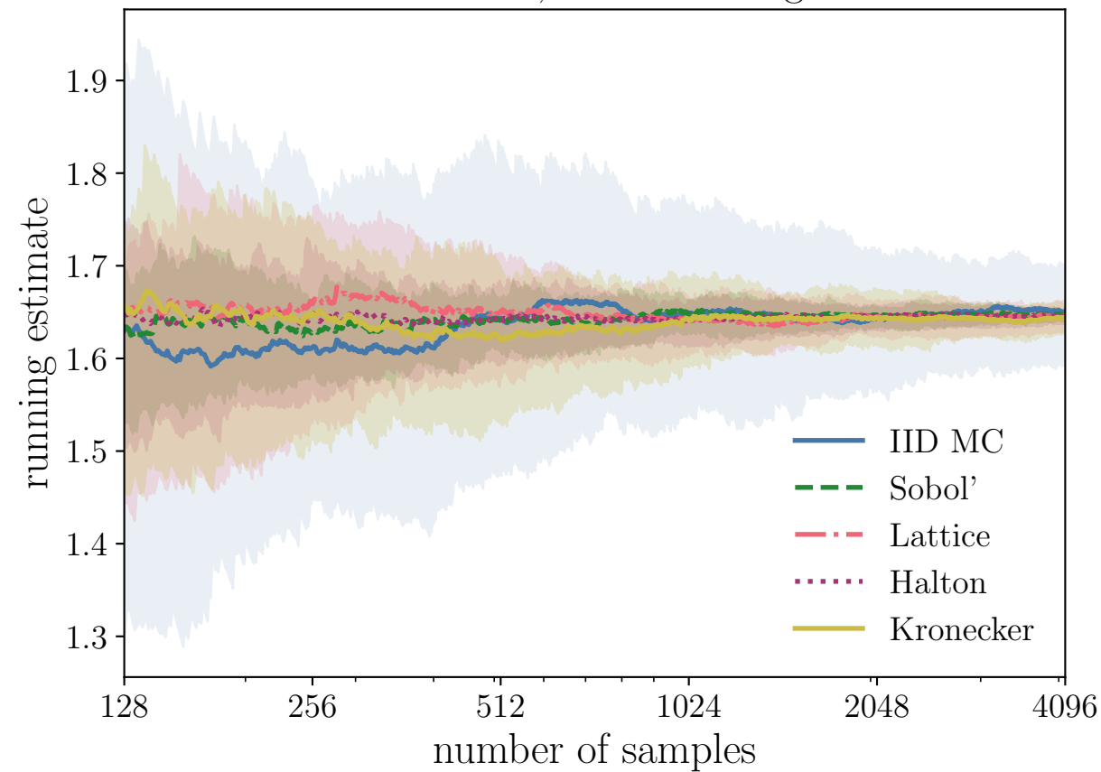
Posterior Gaussian, PCA: running estimates
