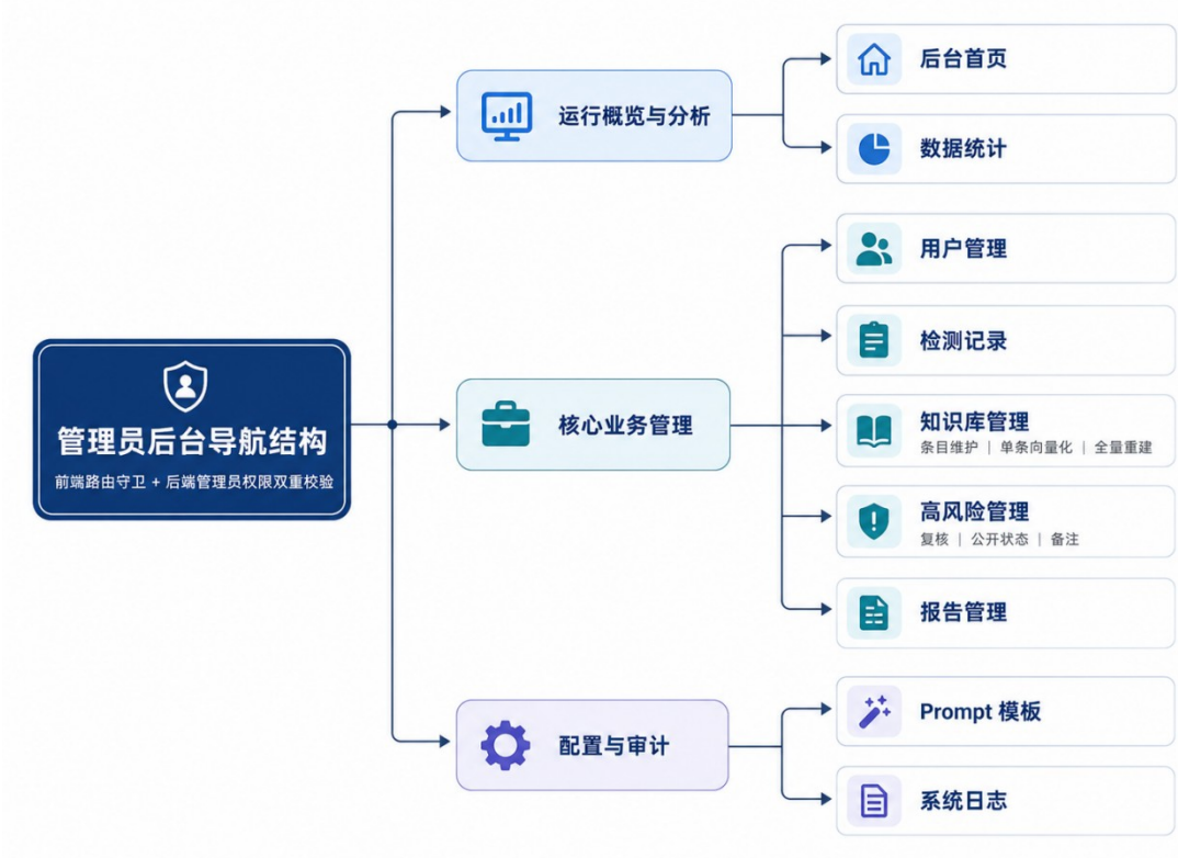
图 4-10 管理员端页面结构图
