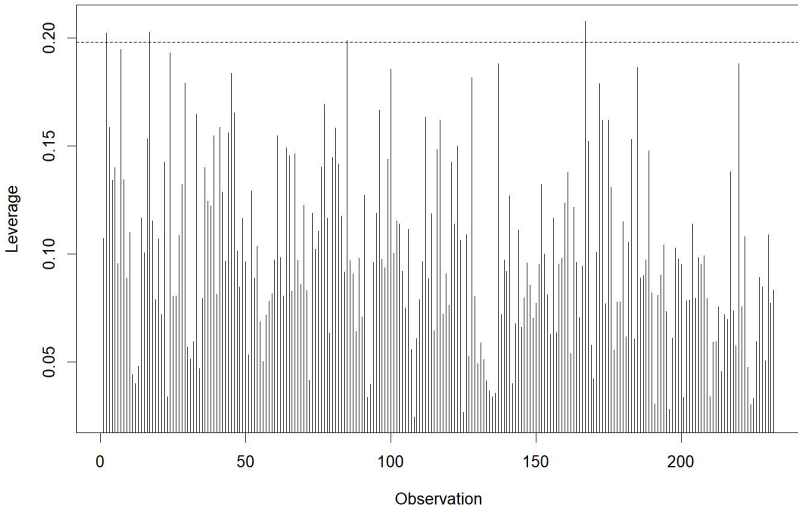
Leverage values
