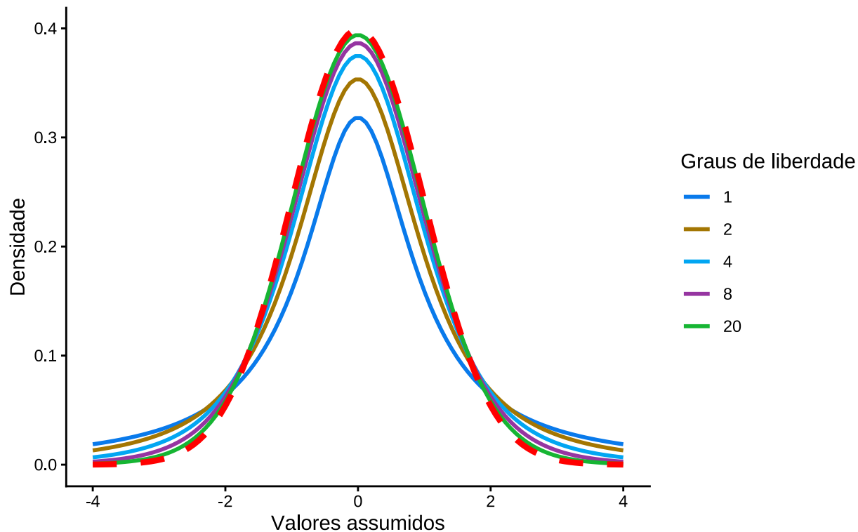
Distribuição t sob diferentes graus de liberdade e sua aproximação à Normal padronizada)
