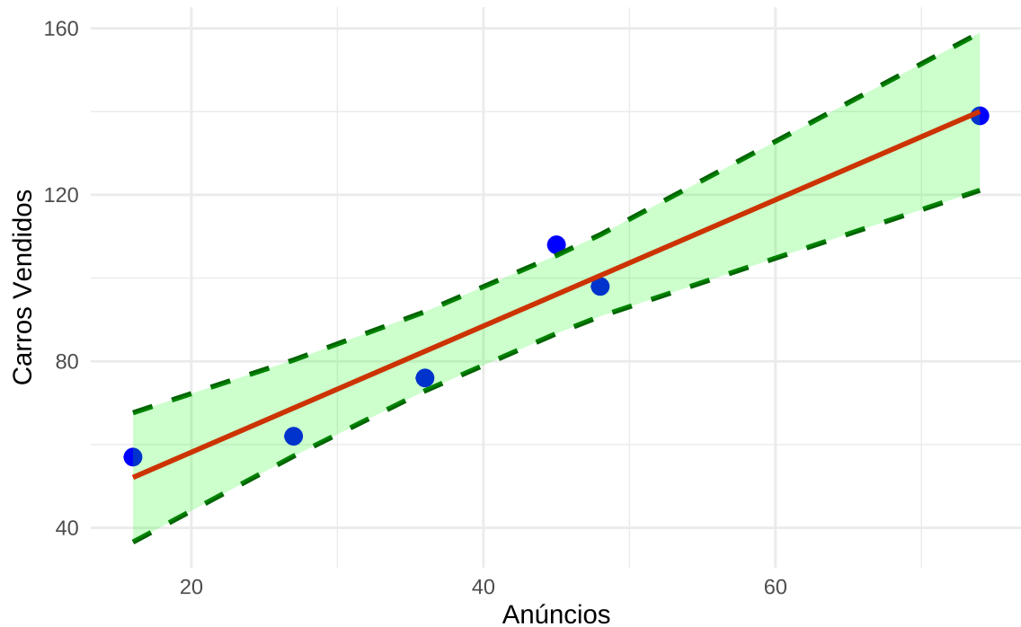
Regressão Linear com Bandas de Confiança (95%)
